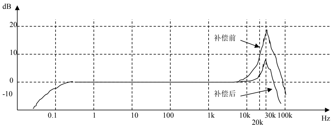
图 7 幅值频率特性曲线高频补偿前后比较
